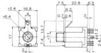
K3610A /B /C /D /E 3.5mm Phone jack
