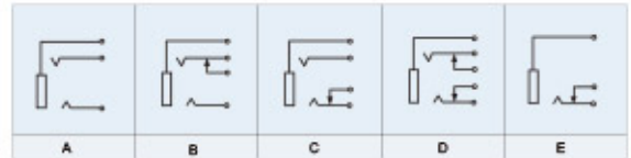
K3610A /B /C /D /E 3.5mm Phone jack
